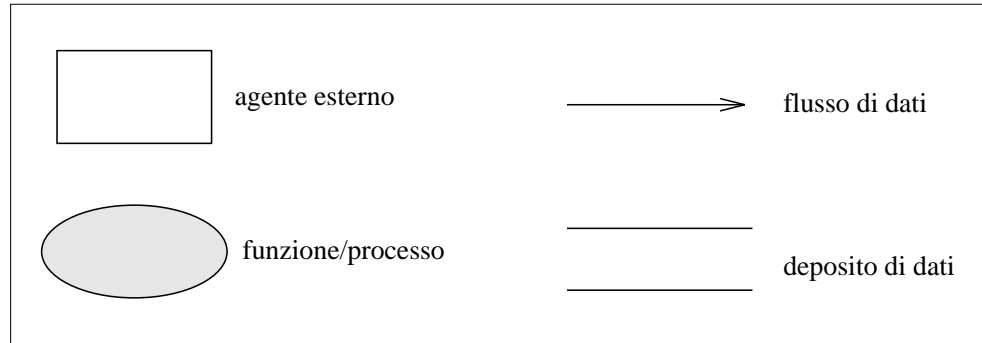
Figura 4.5: Elementi di un DFD
