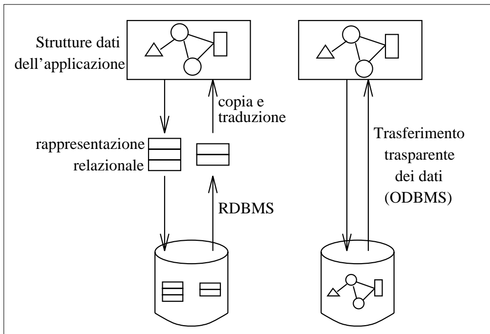
Figura 3.2: Confronto tra architetture di DBMS
