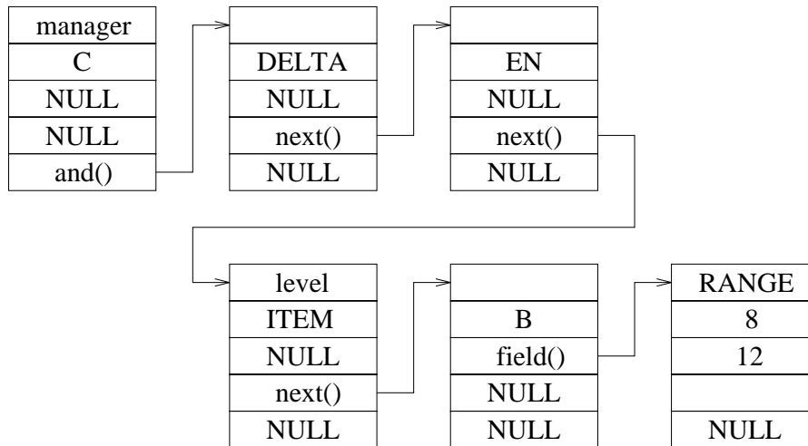
Figura 4.10: descrizione del tipo tmanager
