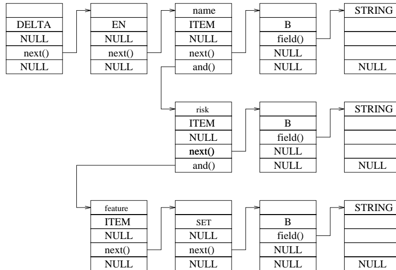
Figura 4.11: descrizione del tipo material
