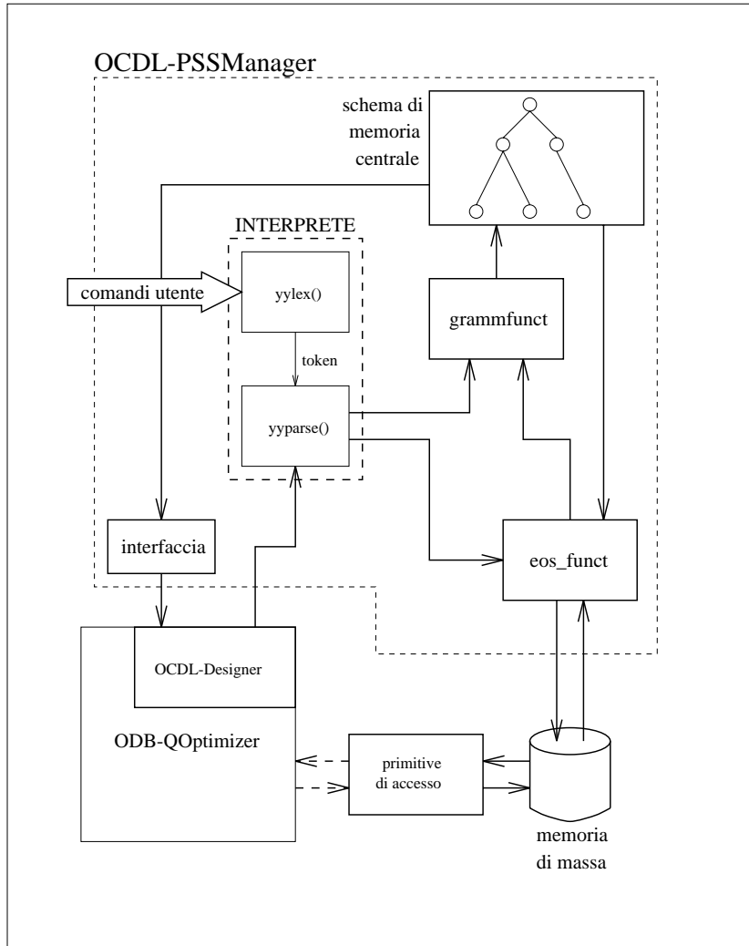
Figura 4.4: Architettura di OCDL-PSSManager
