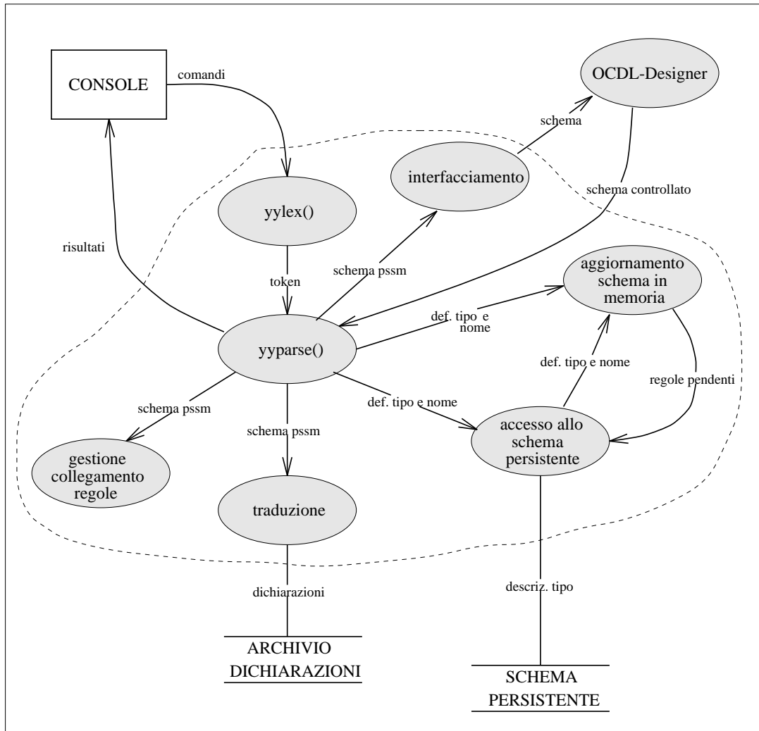
Figura 4.7: Visione dettagliata di OCDL-PSSManager
