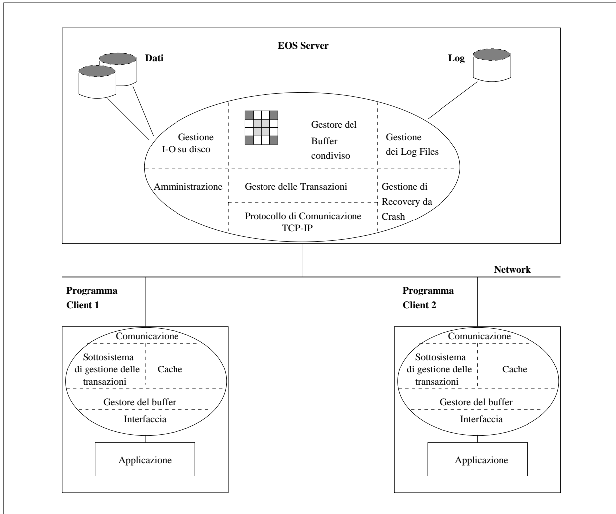
Figura 2.1: Architettura Client-Server di EOS
