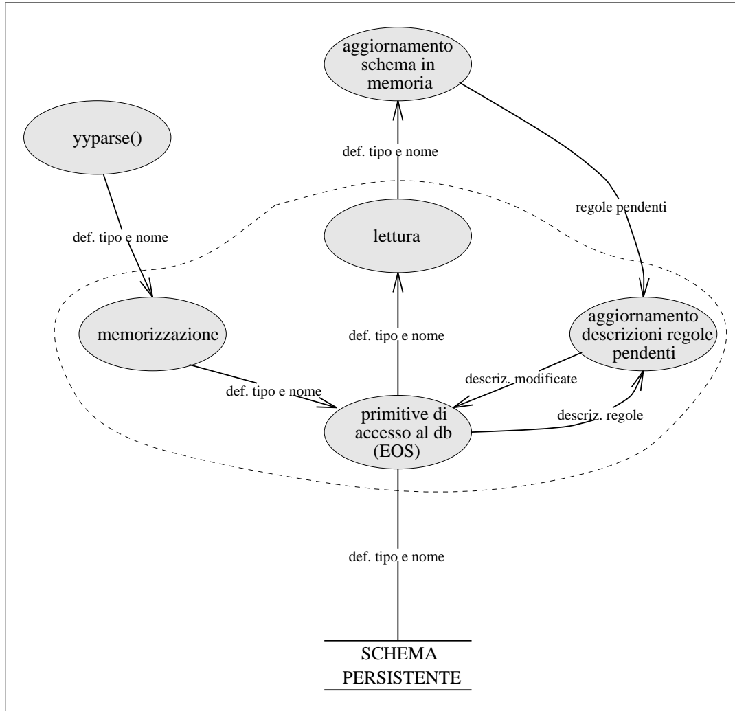
Figura 4.9: Aggiornamento dello schema persistente
