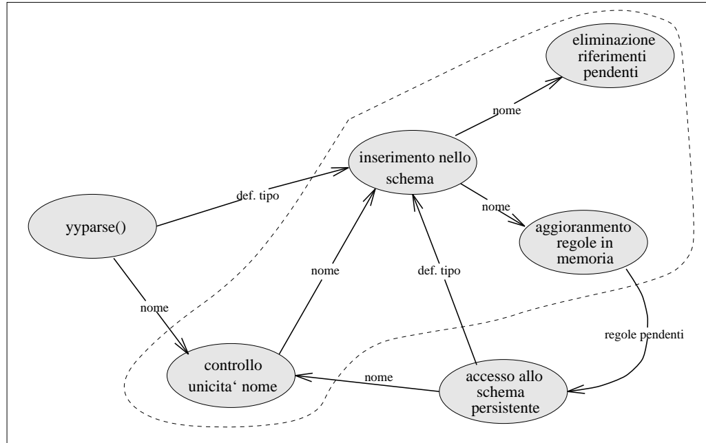
Figura 4.8: Aggiornamento dello schema in memoria centrale
