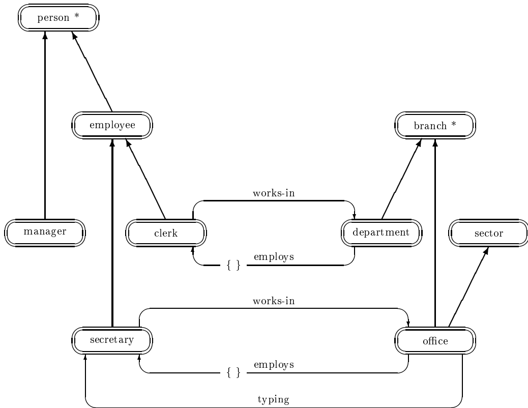
Figura 3.1: Gerarchia delle classi relativa alla struttura organizzativa di una società
