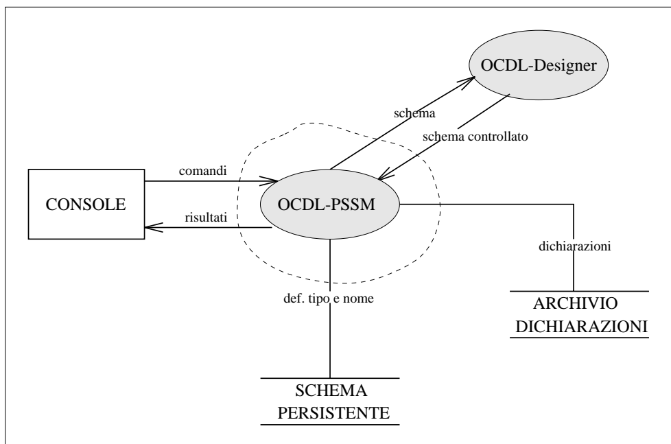
Figura 4.6: architettura funzionale del sistema con OCDL-PSSManager e OCDL-Designer
