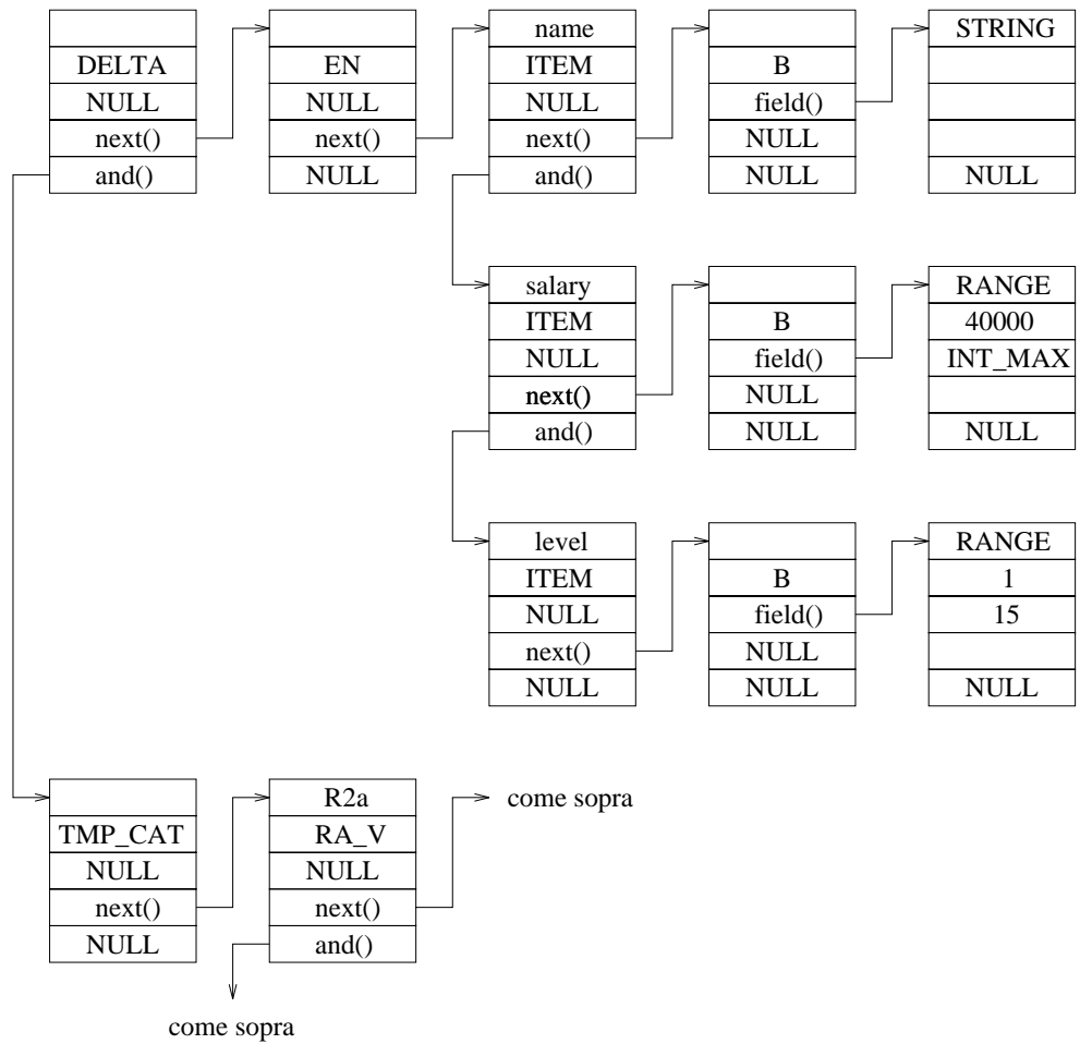
Figura 4.13: esempio di collegamento tipo-regola
