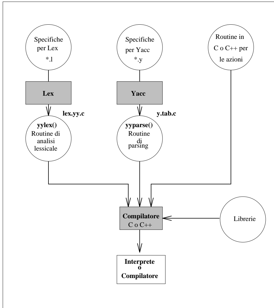
Figura 4.1: Interazione fra lex e yacc
