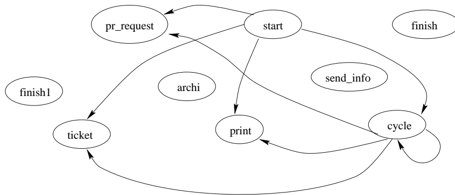
Figura 8.3: Nodi e archi del grafo TG_R
