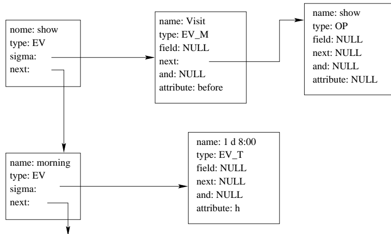
Figura 7.4: Struttura in memoria degli eventi
