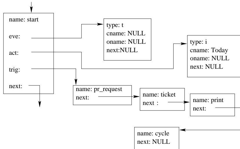
Figura 8.1: Esempio di memorizzazione di una regola per l'algoritmo di terminazione
