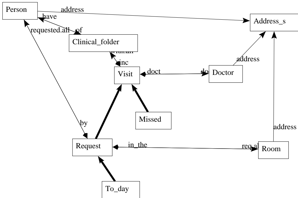
Figura 6.1: Schema dell'esempio in ODB-Tools
