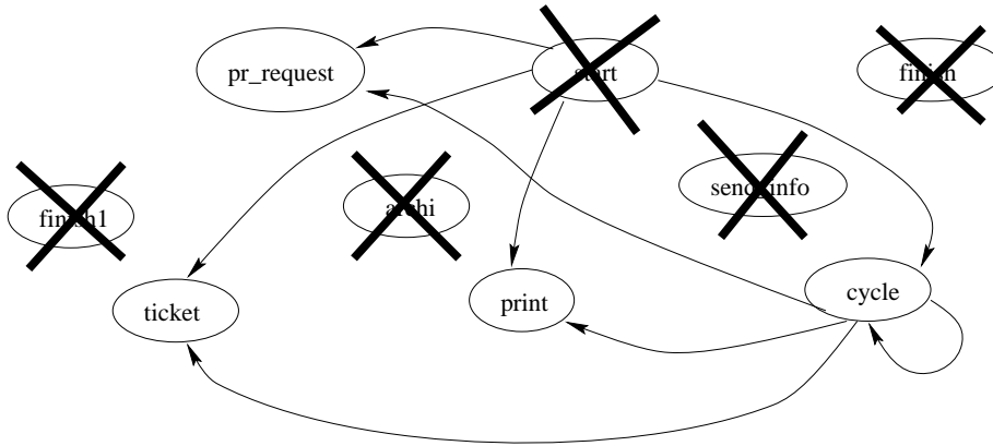
Figura 8.4: Nodi e archi del grafo TG_R dopo l'esecuzione dell'algoritmo di riduzione
