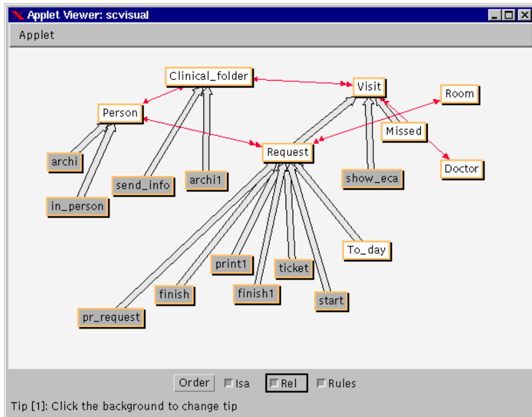
Figura 6.2: Schema CLINIC con regole attive
