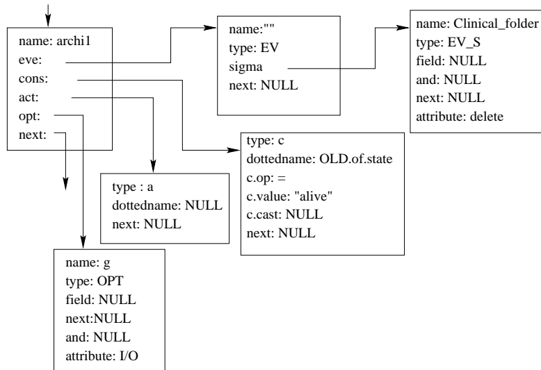
Figura 7.5: Struttura in memoria delle regola attiva archil
