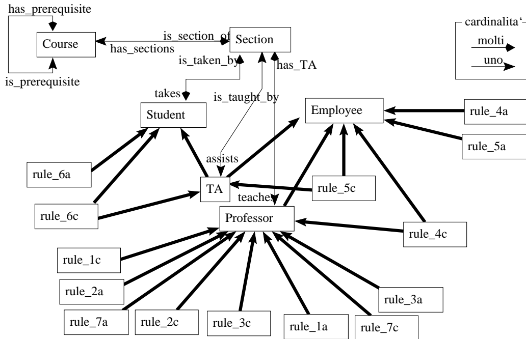
Figura 4.4: Schema dell'esempio con indicazione esplicita delle rules
