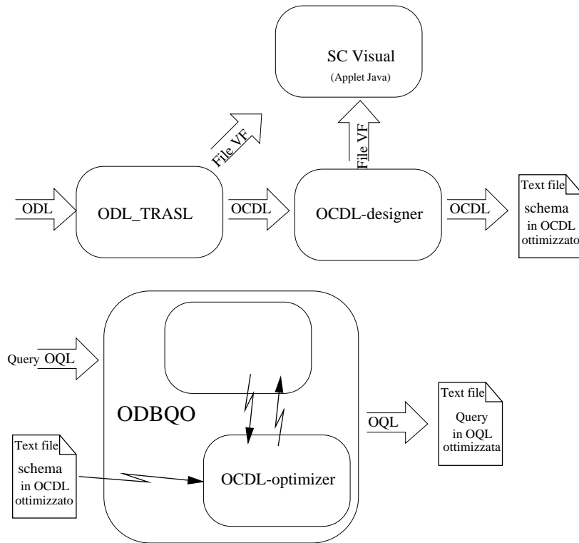
Figura 2.3: Componenti ODB-Tools
