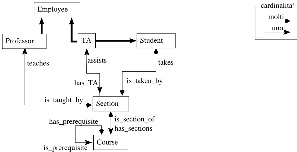
Figura 2.2: Schema dell'esempio
