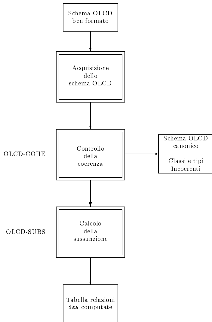
Figura 2.4: Architettura funzionale di OCDL-Designer
