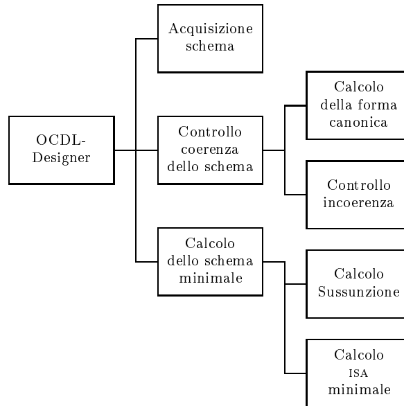
Figura 2.5: Struttura del programma OCDL-Designer
