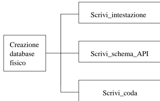
Figura 4.2: Struttura del modulo per la creazione del database fisico in UNISQL/X
