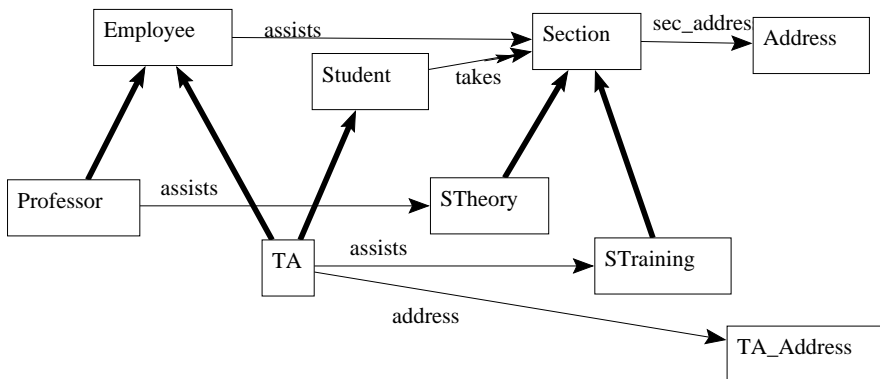
Figura 2.1: Rappresentazione grafica dello schema Università
