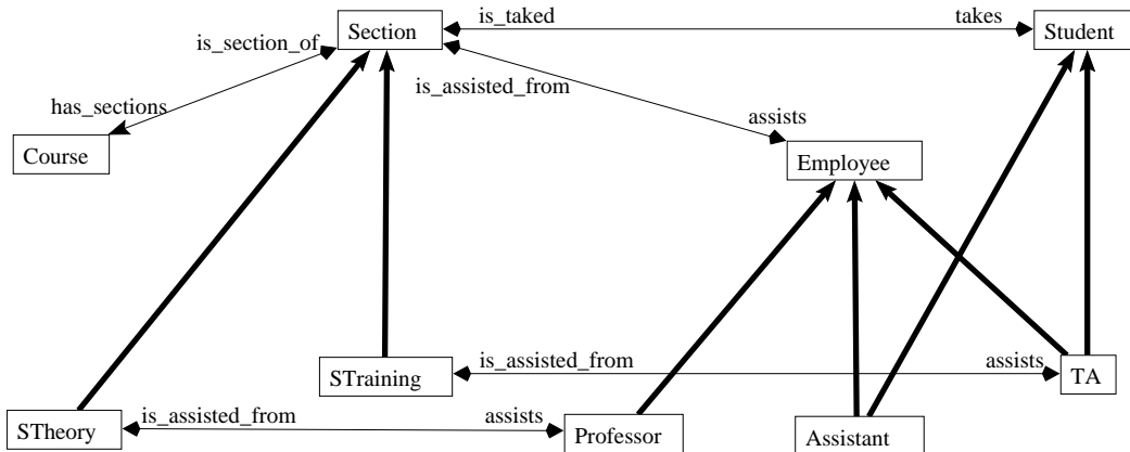
Figura A.2: Schema del database di un' università
