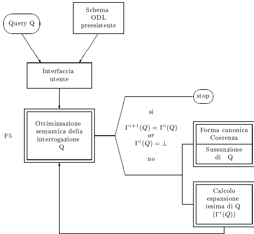
Figura 5.5: Architettura funzionale di ODB-QOptimizer
