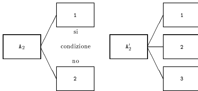
Figura 5.8: Esempio di chiamate in alternativa
