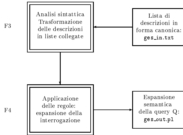
Figura 5.4: Architettura funzionale di GES
