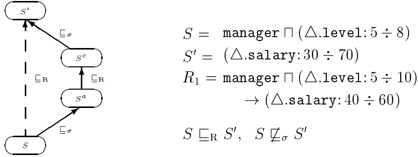
Figura 4.1: Relazione di sussunzione forzata mediante una regola.
