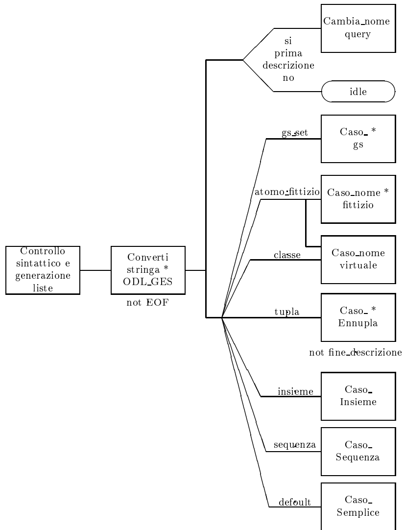
Figura 5.14: Sottomodulo "Controllo sintattico e generazione liste"
