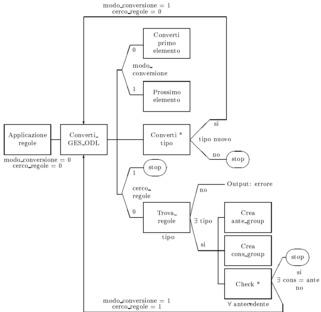
Figura 5.16: Modulo "Applicazione delle regole"
