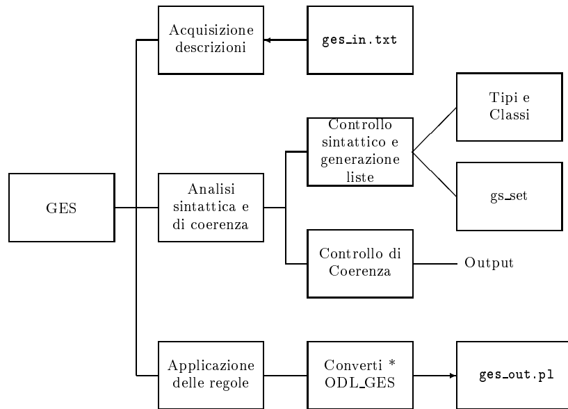
Figura 5.11: Struttura del programma GES
